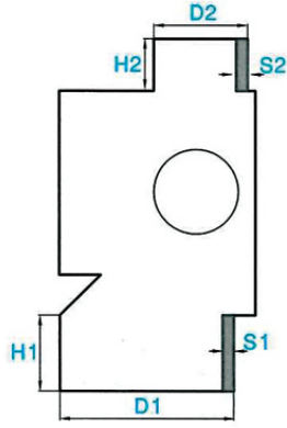
Floor trap 7 cm / بيبة 7 سم
